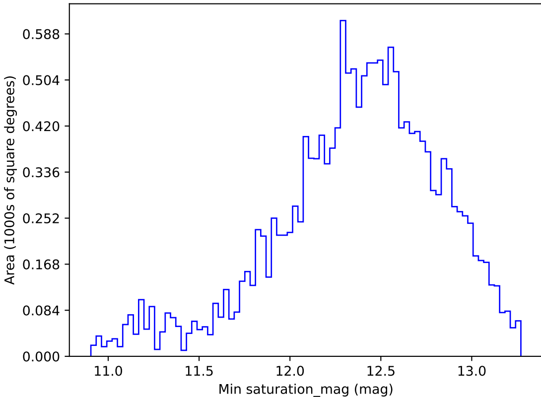
baseline_v3.3_10yrs WFD i band: Min saturation_mag
