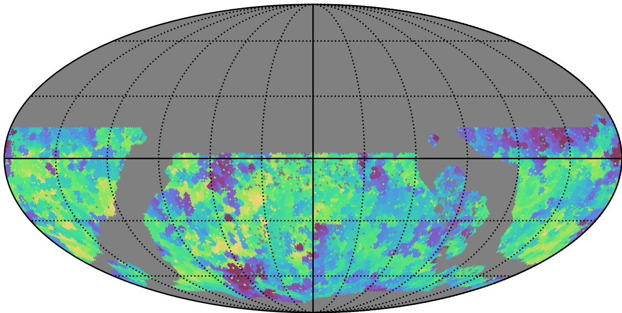
baseline_v3.3_10yrs WFD g band: Min saturation_mag
