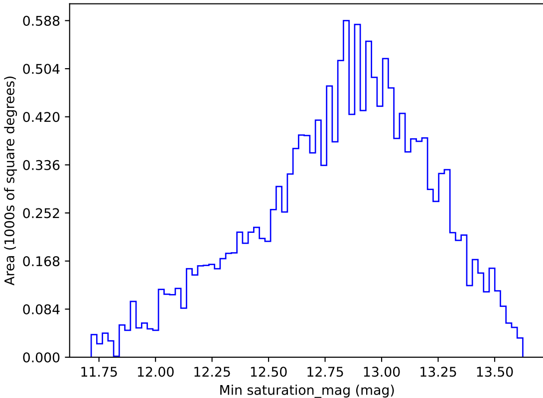
baseline_v3.3_10yrs WFD g band: Min saturation_mag
