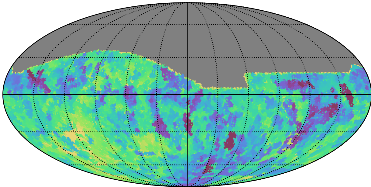
baseline_v3.3_10yrs All sky z band: Min saturation_mag
