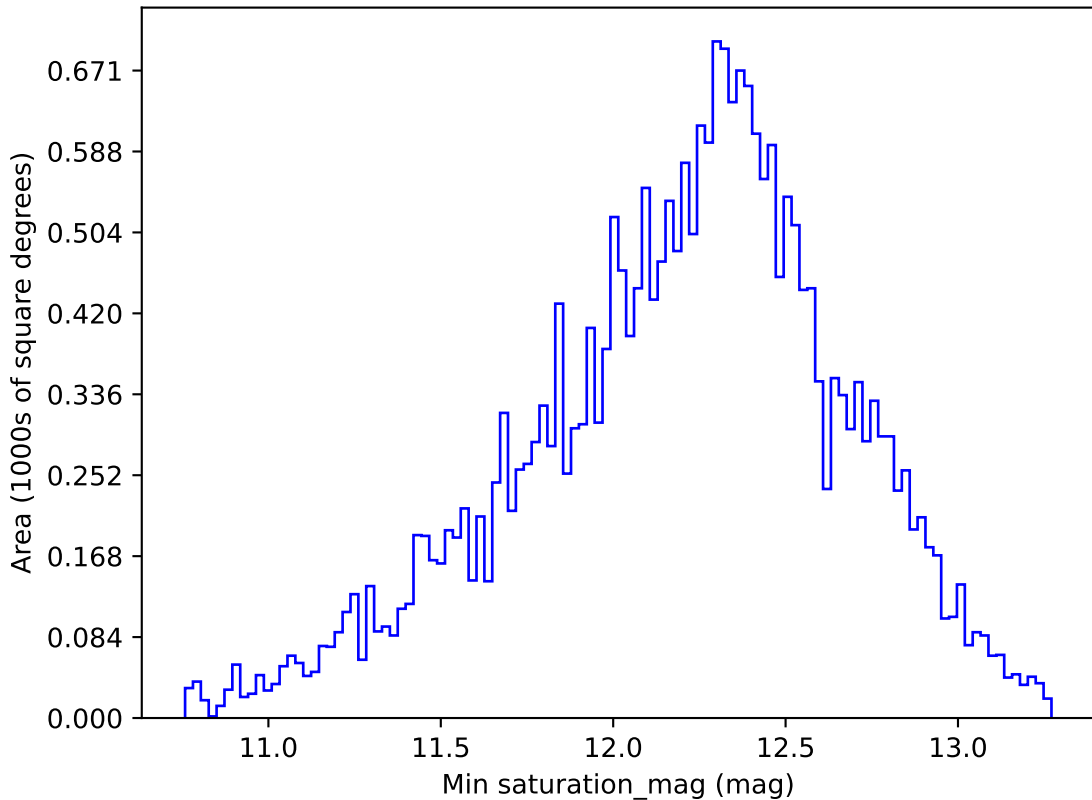
baseline_v3.3_10yrs All sky z band: Min saturation_mag
