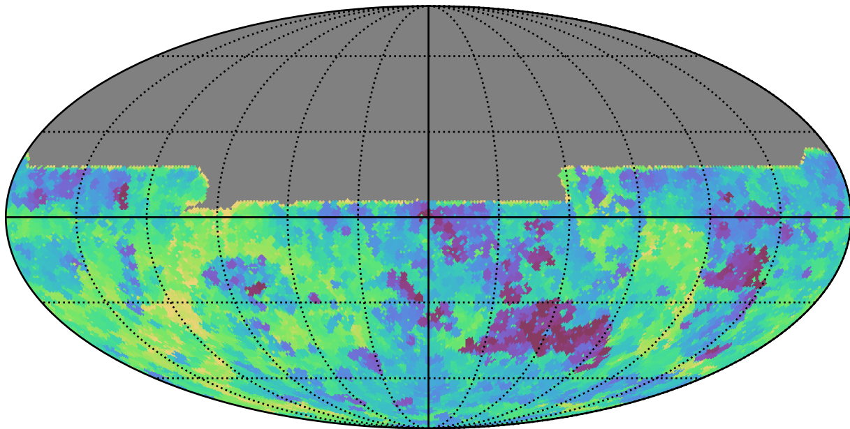
baseline_v3.3_10yrs All sky y band: Min saturation_mag
