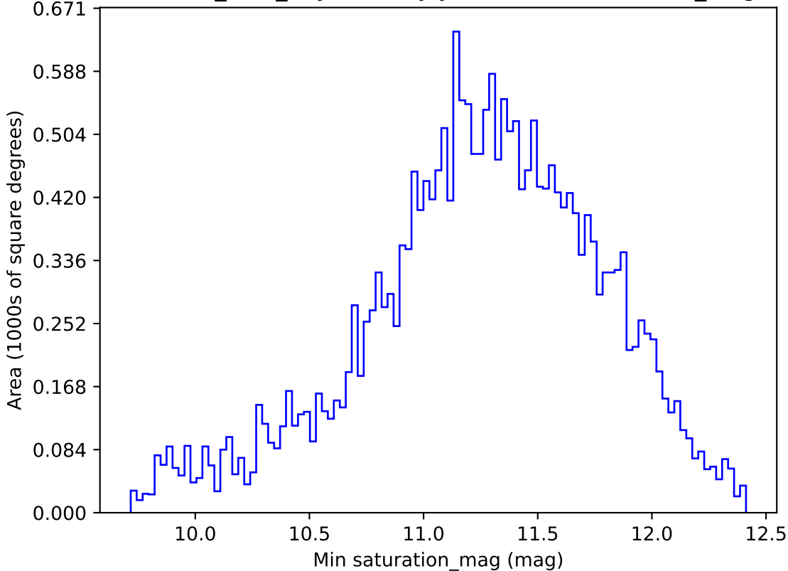
baseline_v3.3_10yrs All sky y band: Min saturation_mag
