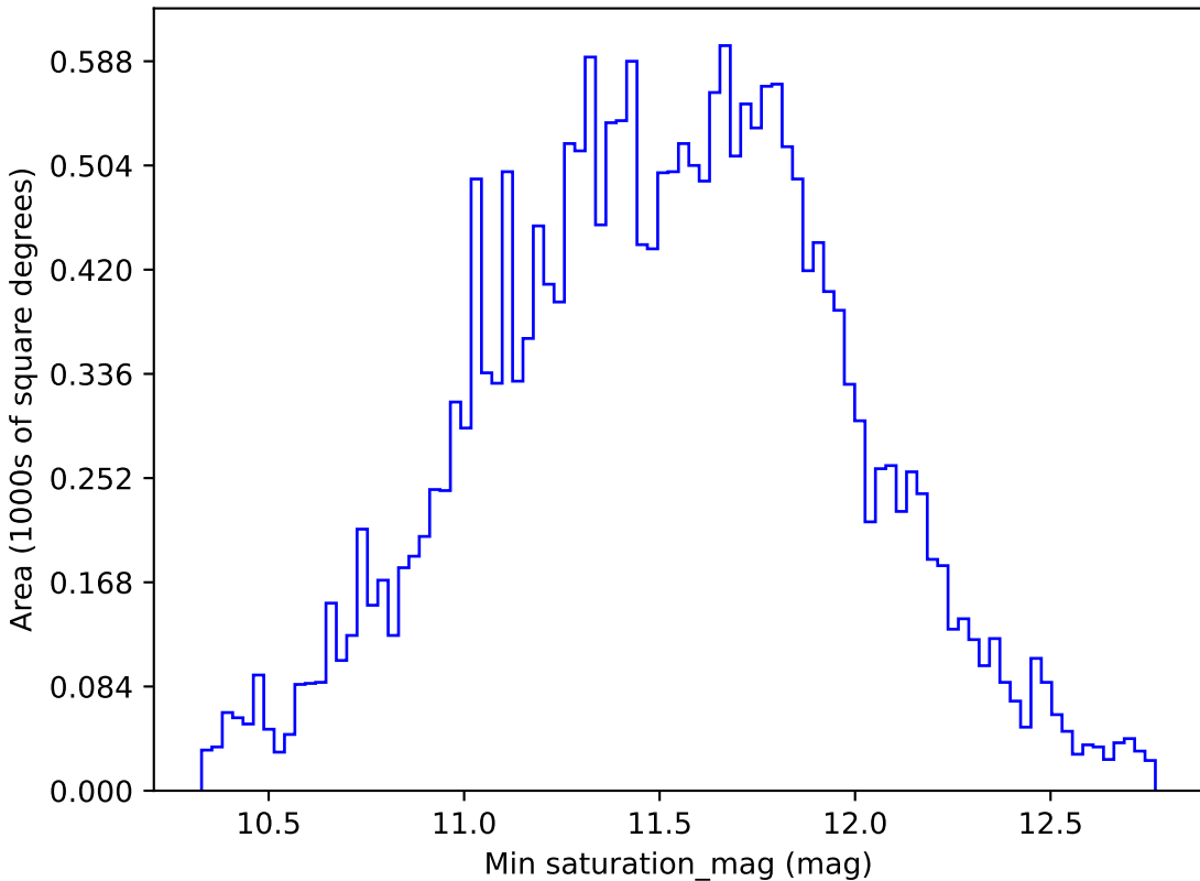
baseline_v3.3_10yrs All sky u band: Min saturation_mag
