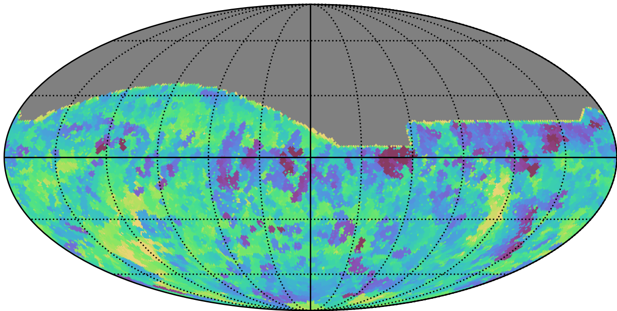
baseline_v3.3_10yrs All sky r band: Min saturation_mag
