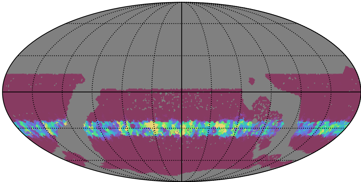
baseline_v3.3_10yrs WFD z band: Min normairmass
