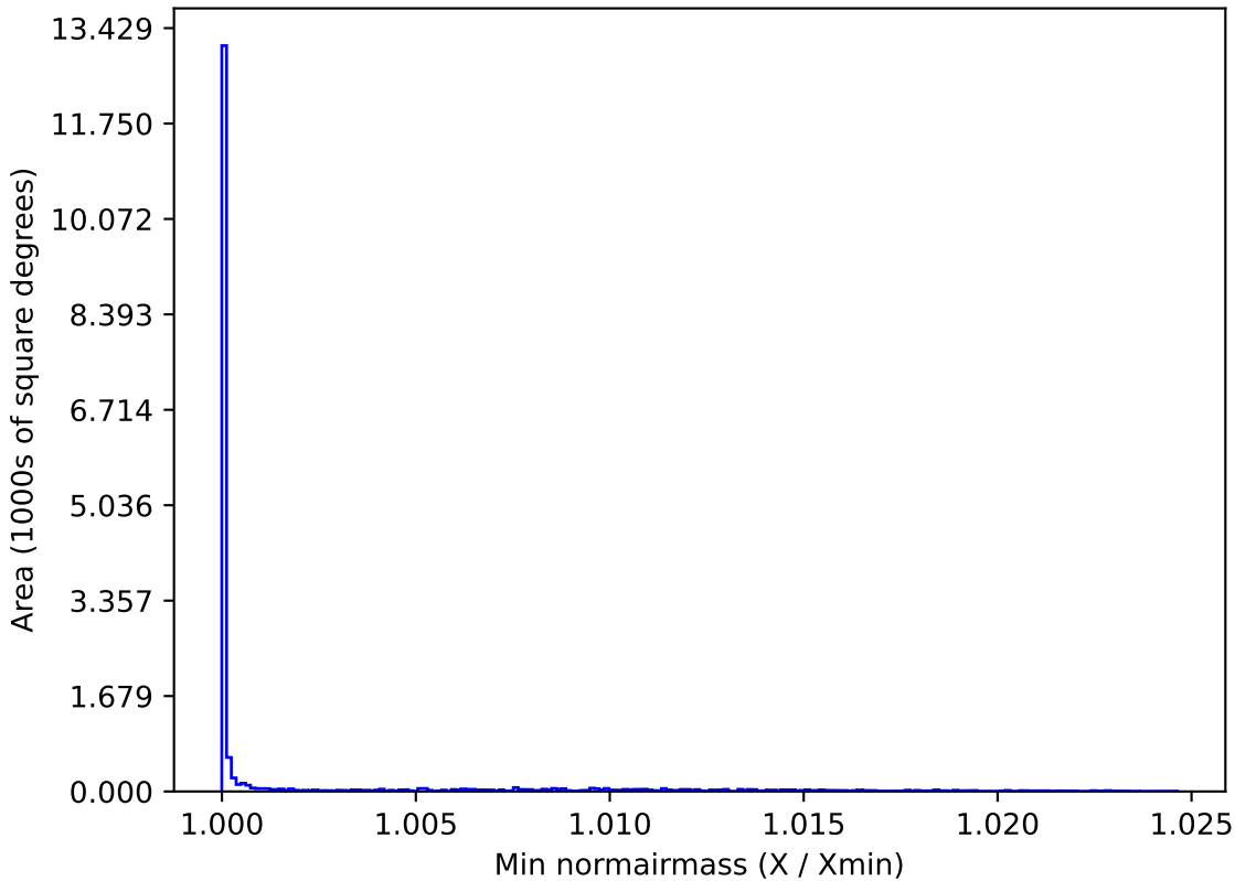
baseline_v3.3_10yrs WFD y band: Min normairmass
