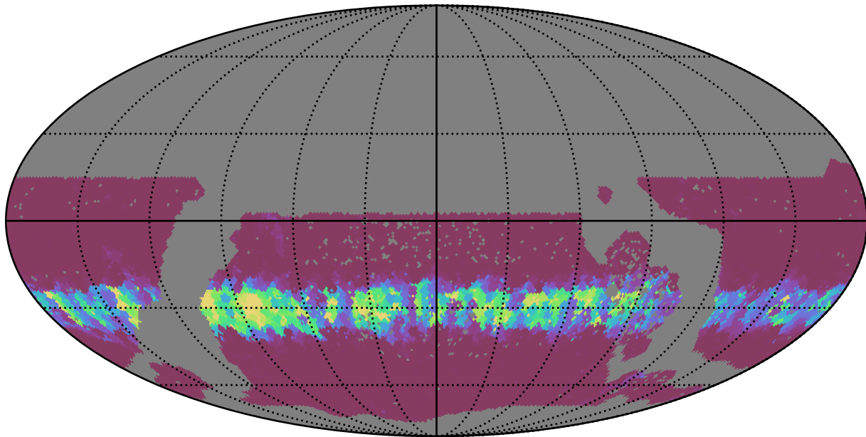
baseline_v3.3_10yrs WFD u band: Min normairmass
