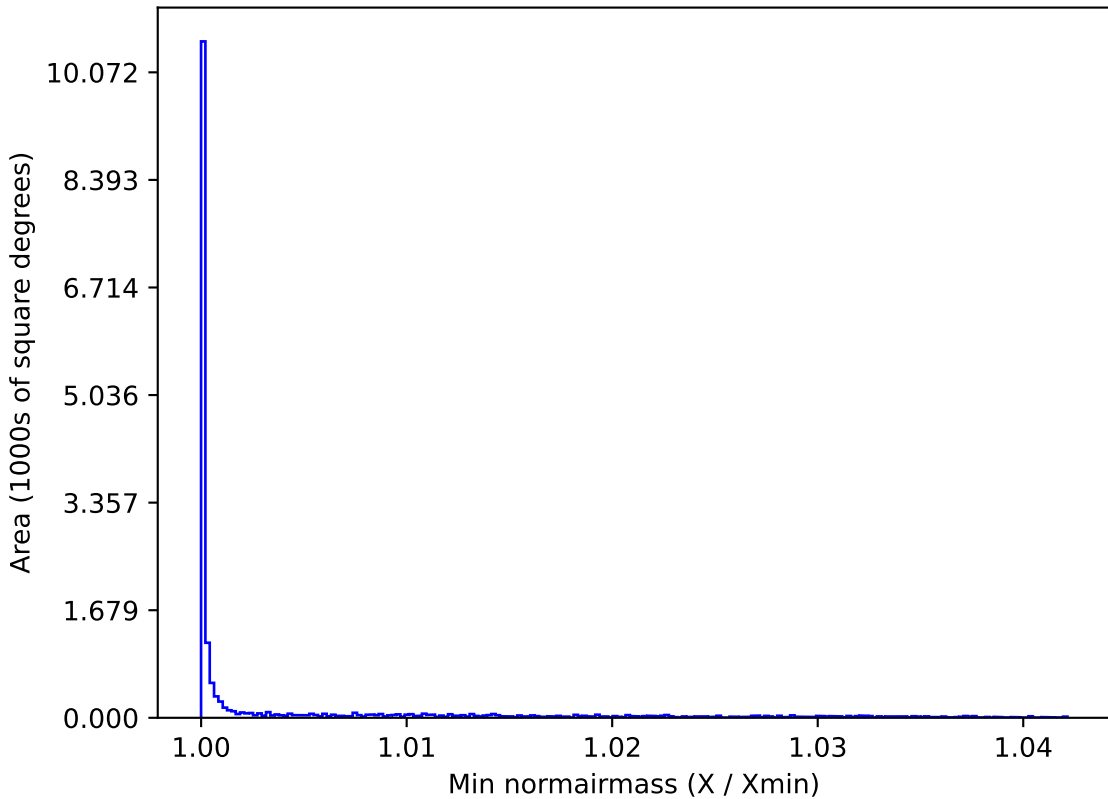
baseline_v3.3_10yrs WFD u band: Min normairmass
