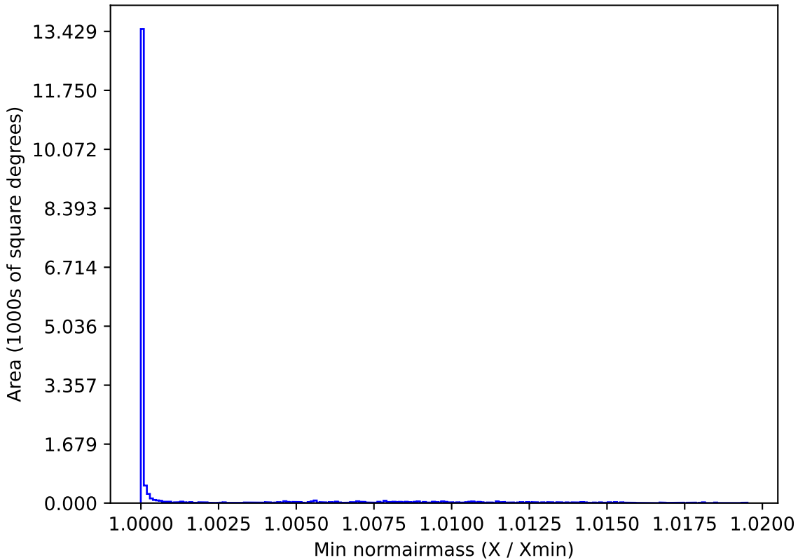
baseline_v3.3_10yrs WFD r band: Min normairmass
