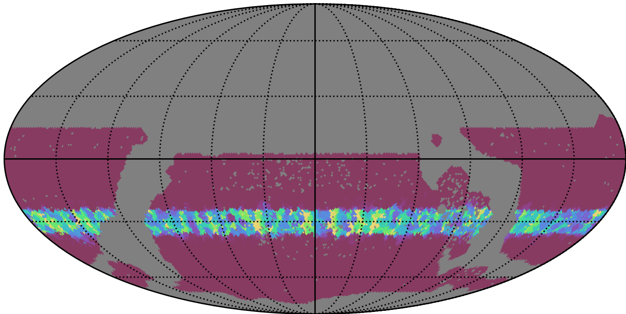
baseline_v3.3_10yrs WFD i band: Min normairmass
