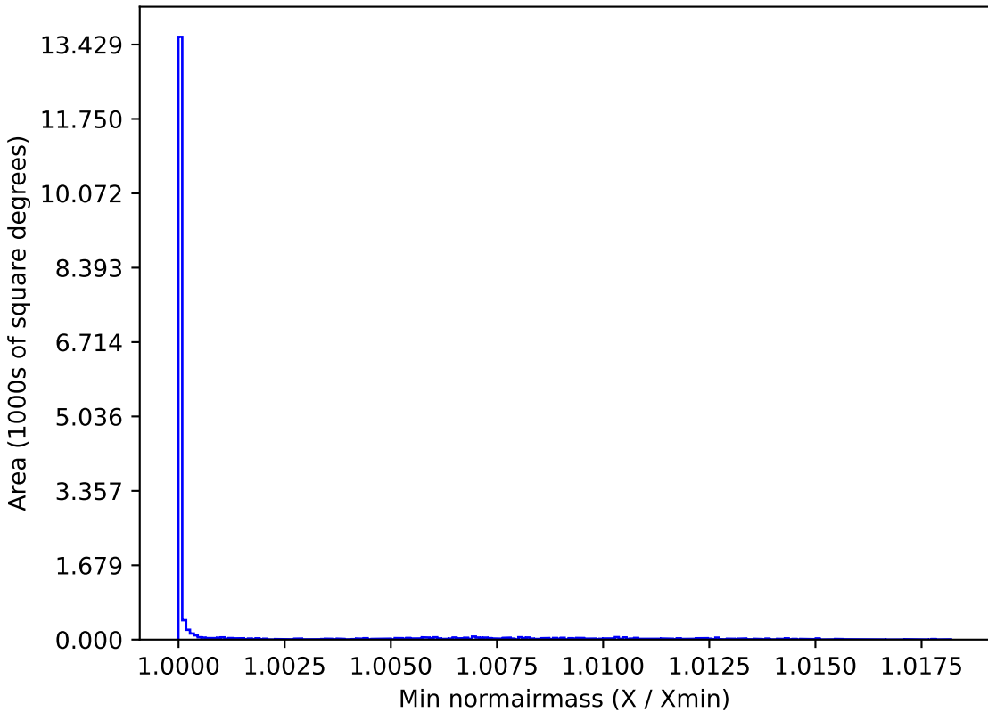
baseline_v3.3_10yrs WFD i band: Min normairmass
