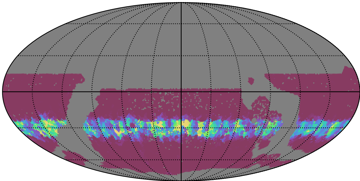
baseline_v3.3_10yrs WFD g band: Min normairmass
