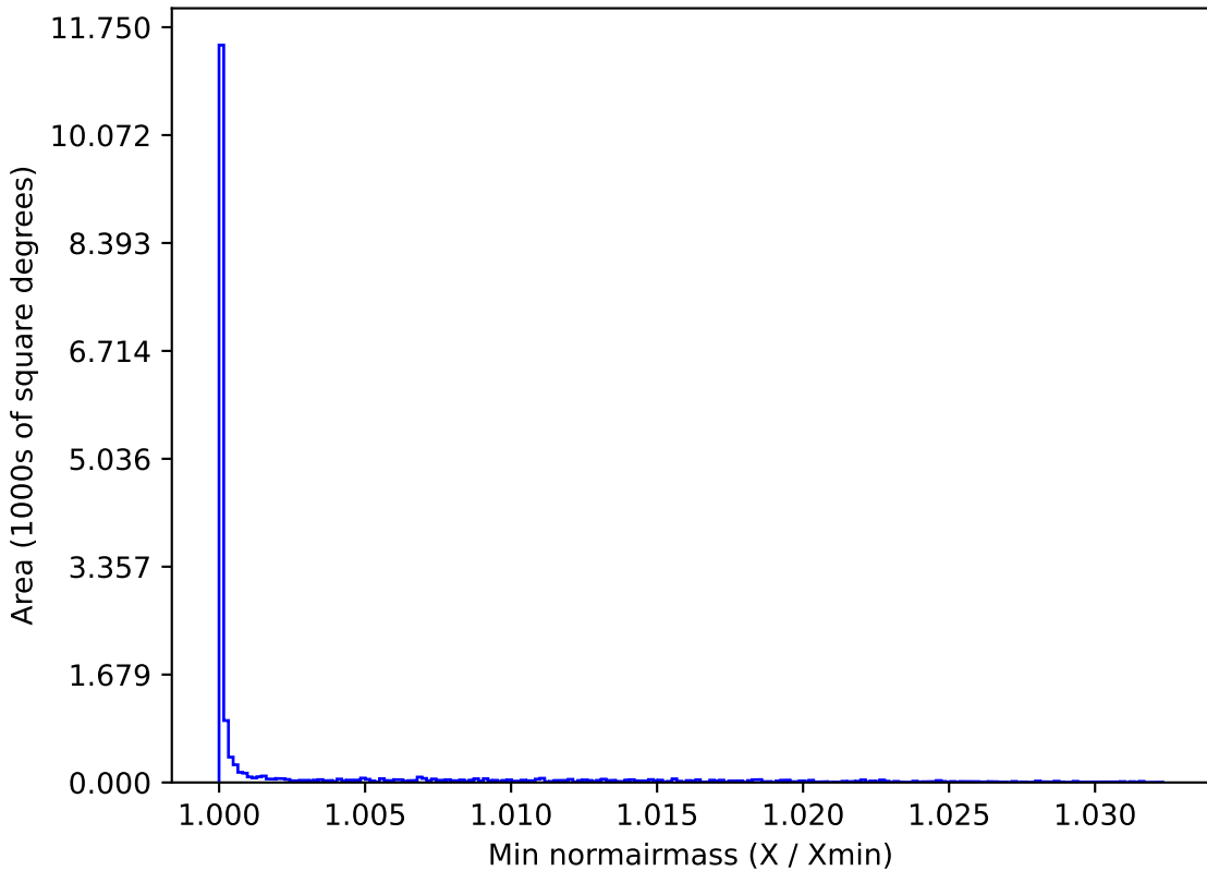
baseline_v3.3_10yrs WFD g band: Min normairmass
