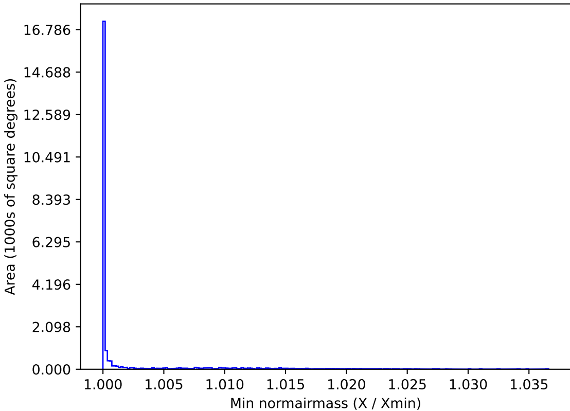
baseline_v3.3_10yrs All sky y band: Min normairmass
