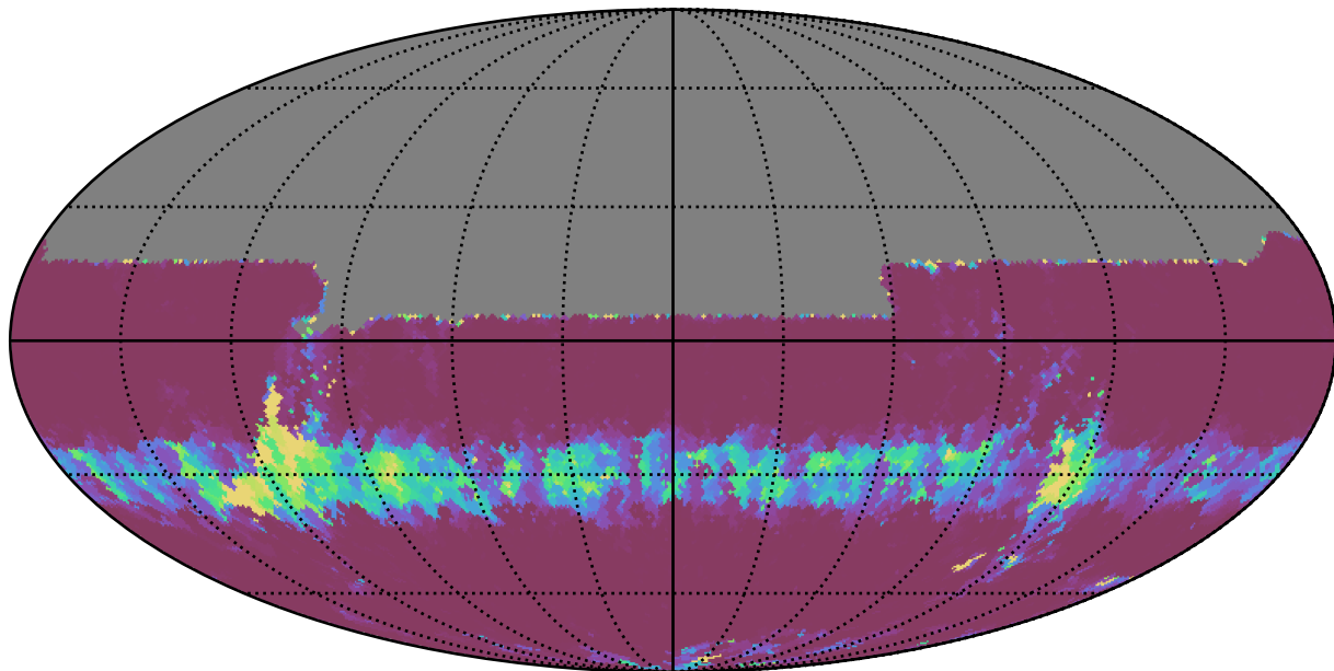
baseline_v3.3_10yrs All sky u band: Min normairmass
