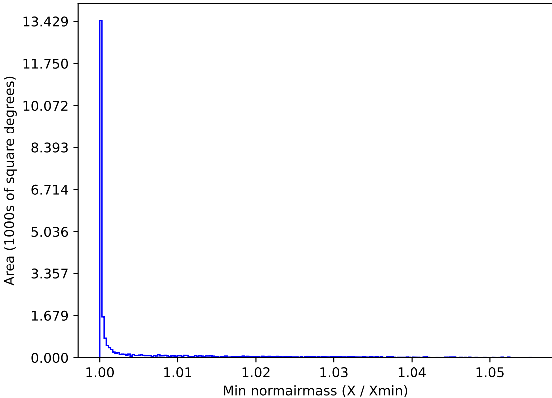
baseline_v3.3_10yrs All sky u band: Min normairmass
