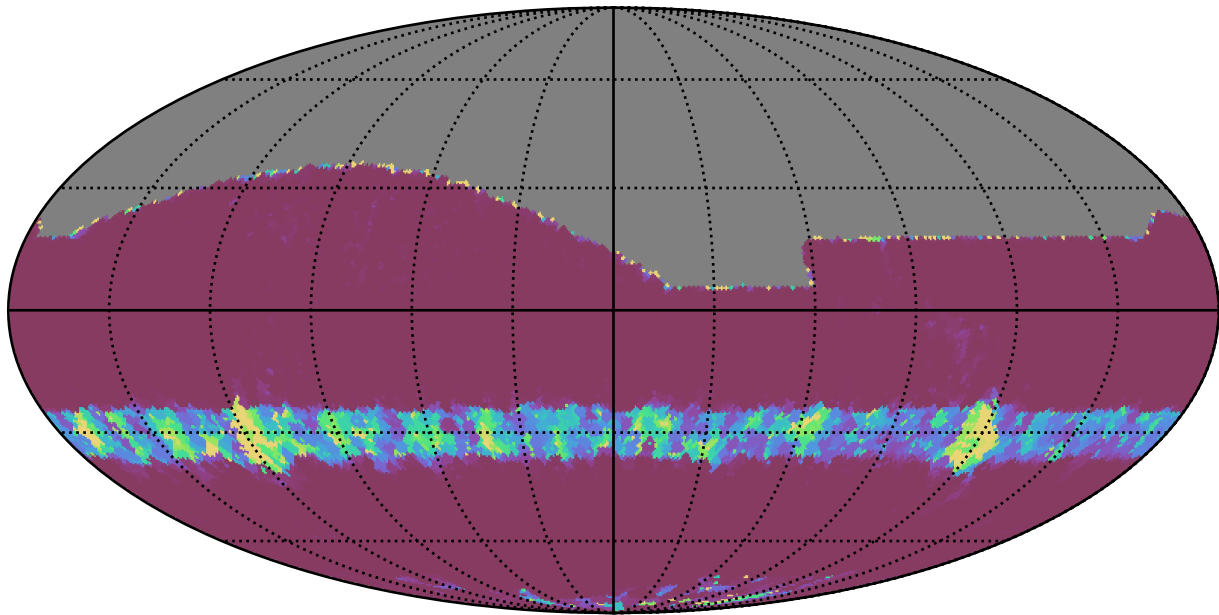
baseline_v3.3_10yrs All sky r band: Min normairmass
