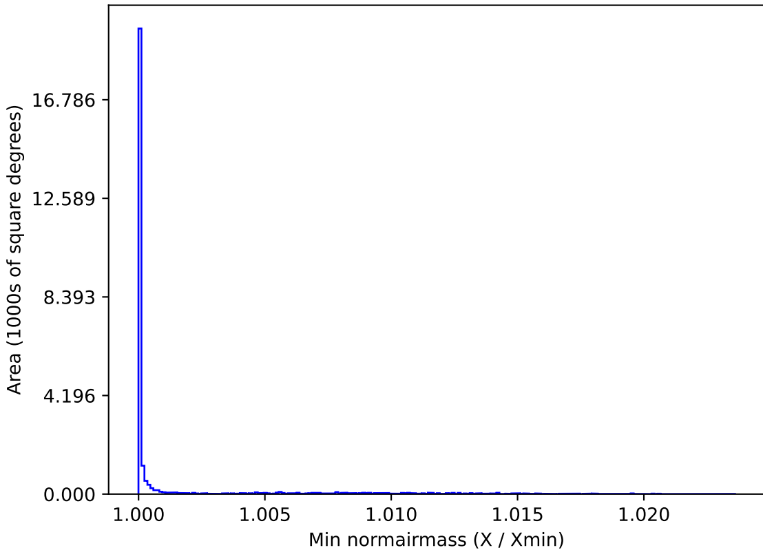
baseline_v3.3_10yrs All sky r band: Min normairmass
