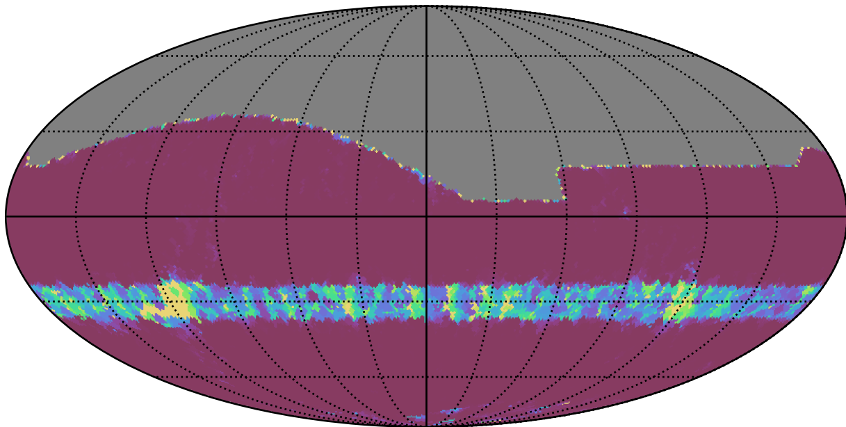
baseline_v3.3_10yrs All sky i band: Min normairmass
