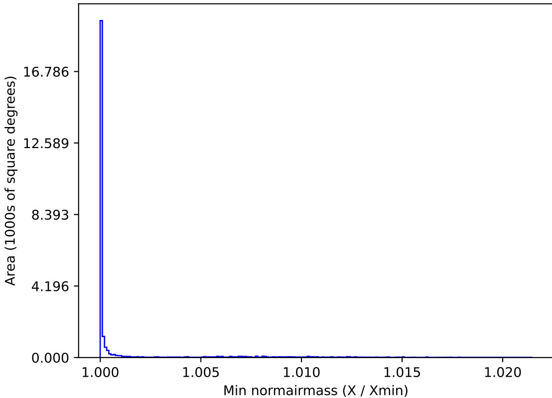
baseline_v3.3_10yrs All sky i band: Min normairmass
