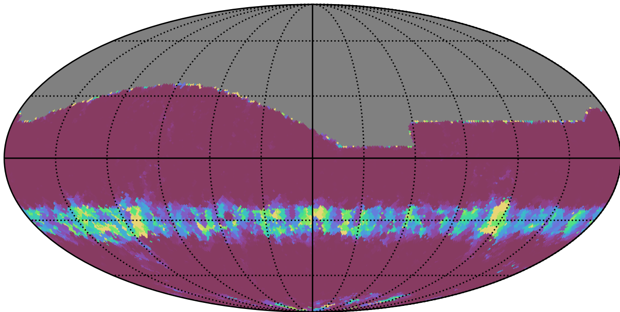
baseline_v3.3_10yrs All sky g band: Min normairmass
