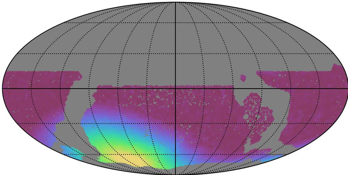
baseline_v3.3_10yrs WFD z band: Min moonDistance
