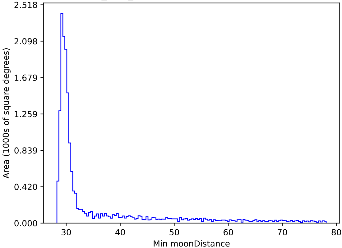
baseline_v3.3_10yrs WFD z band: Min moonDistance
