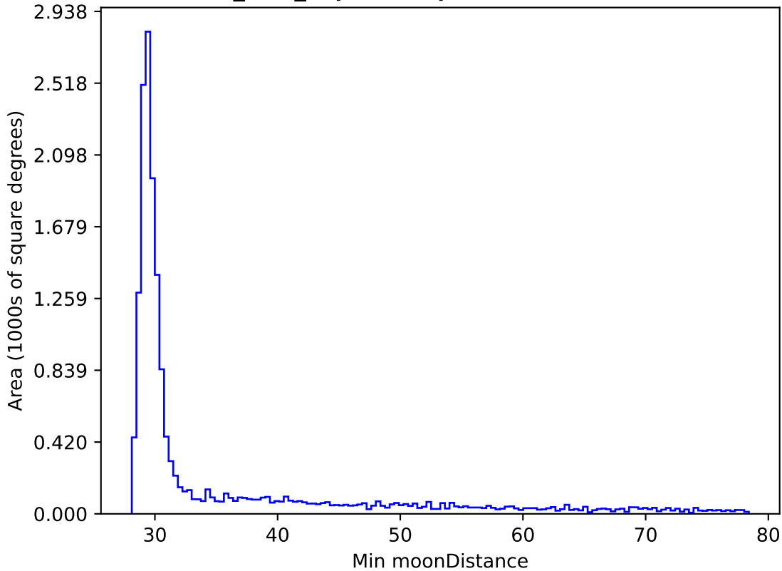
baseline_v3.3_10yrs WFD y band: Min moonDistance
