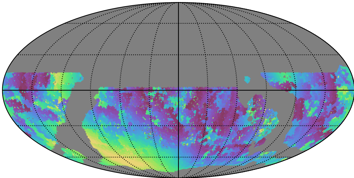
baseline_v3.3_10yrs WFD u band: Min moonDistance
