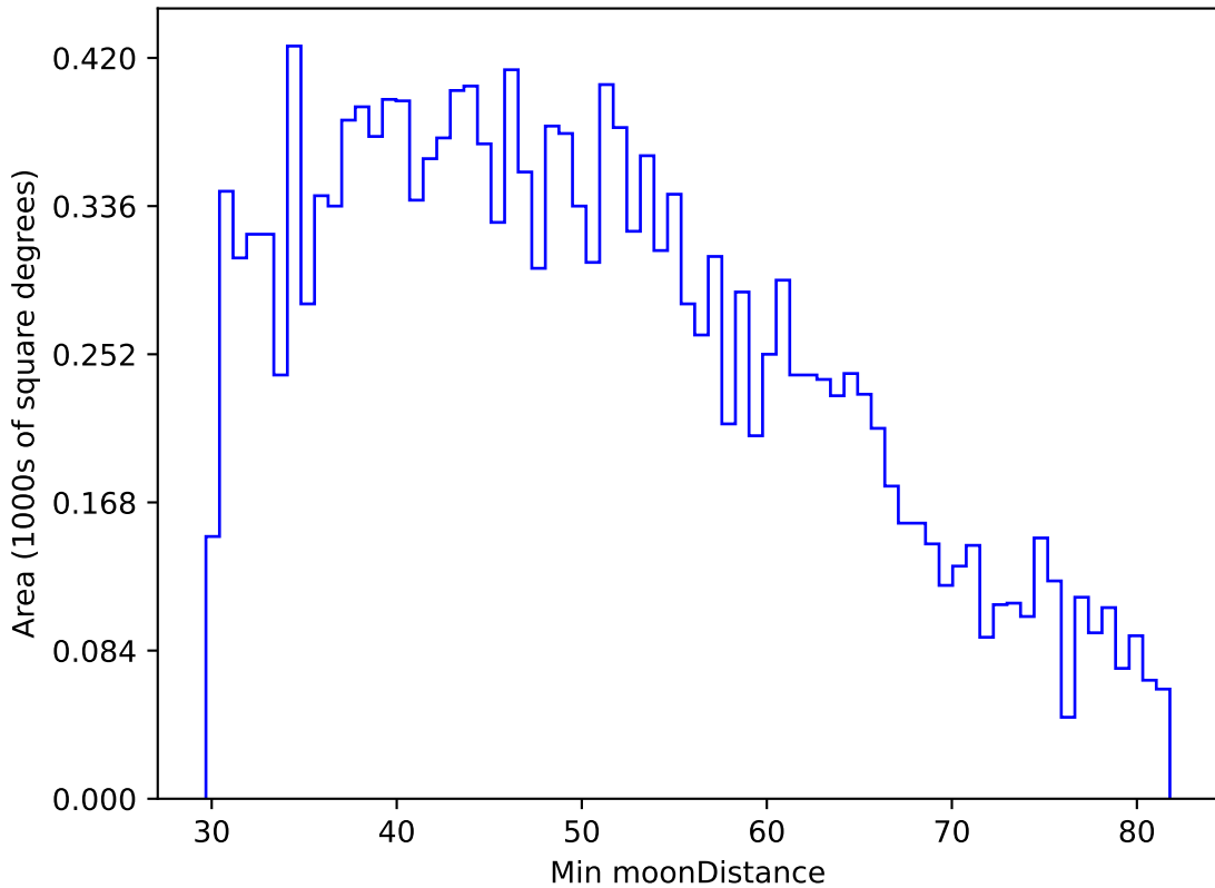
baseline_v3.3_10yrs WFD u band: Min moonDistance
