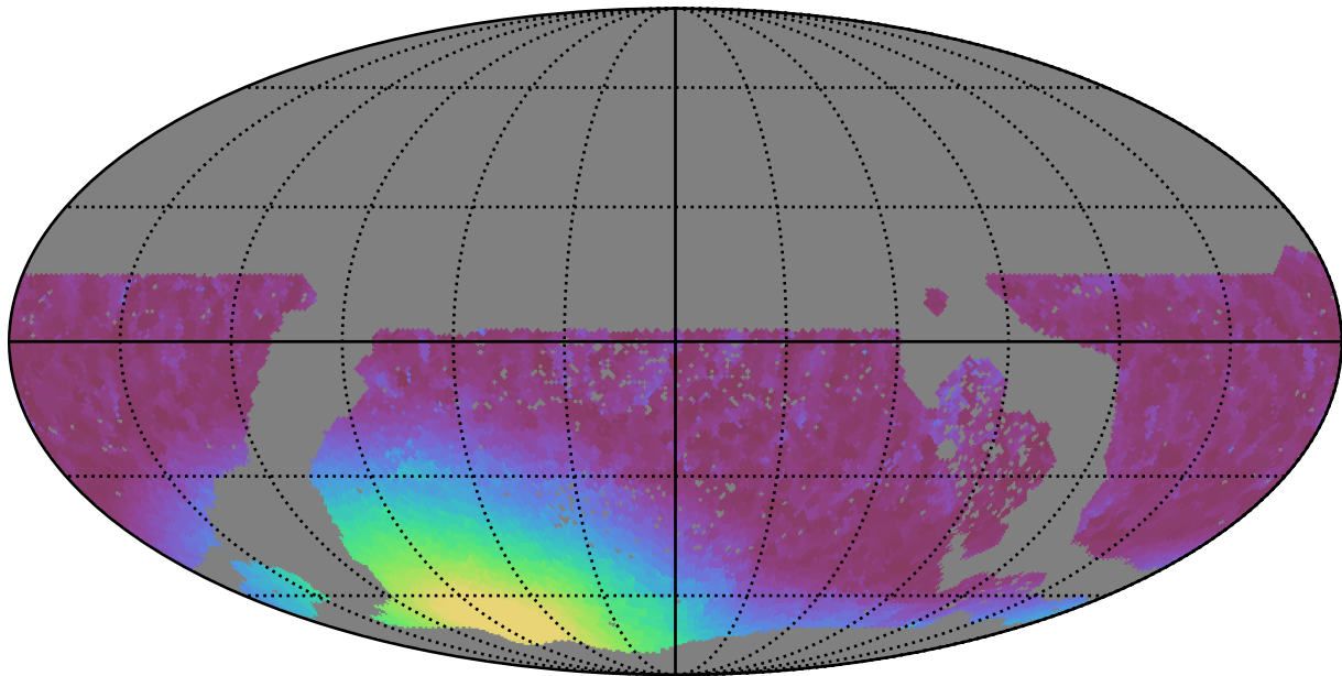
baseline_v3.3_10yrs WFD r band: Min moonDistance
