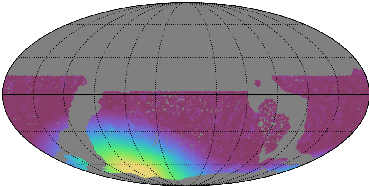
baseline_v3.3_10yrs WFD i band: Min moonDistance
