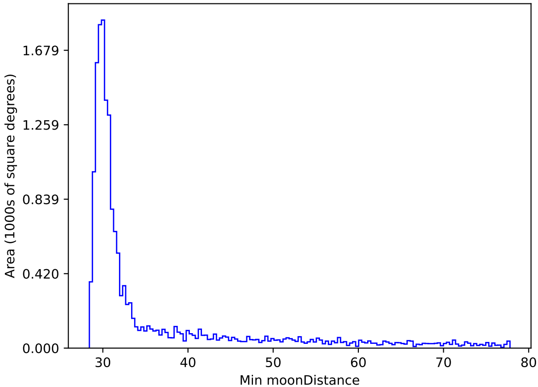
baseline_v3.3_10yrs WFD i band: Min moonDistance
