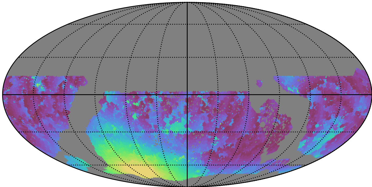
baseline_v3.3_10yrs WFD g band: Min moonDistance
