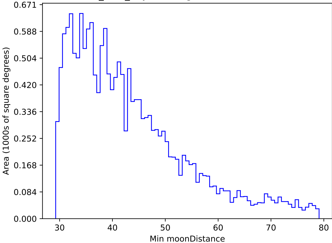
baseline_v3.3_10yrs WFD g band: Min moonDistance
