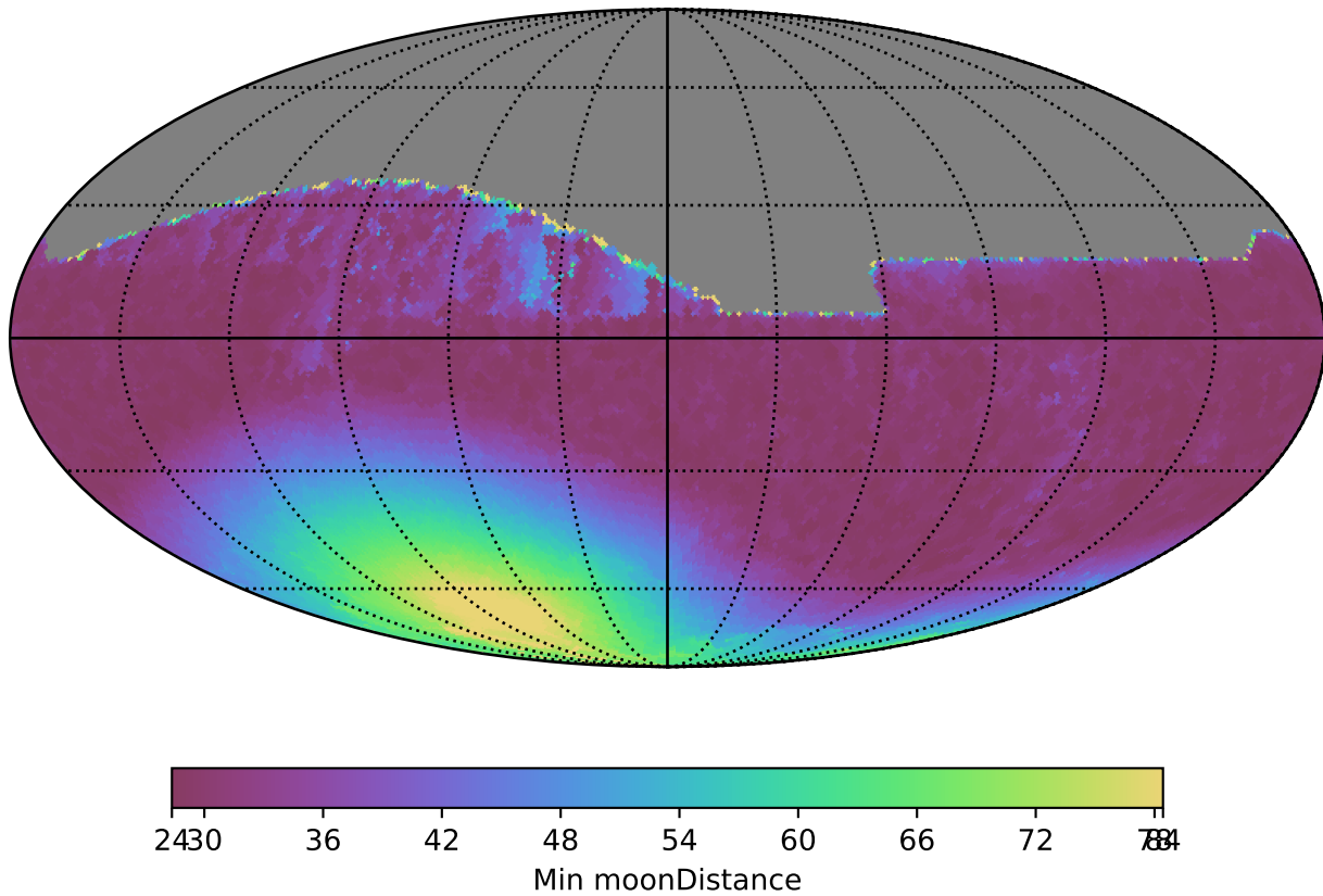
baseline_v3.3_10yrs All sky z band: Min moonDistance
