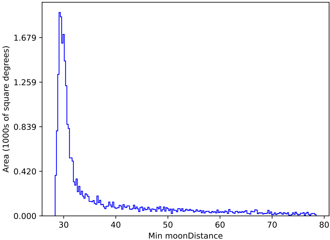
baseline_v3.3_10yrs All sky z band: Min moonDistance
