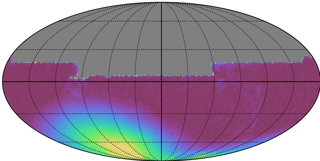
baseline_v3.3_10yrs All sky y band: Min moonDistance
