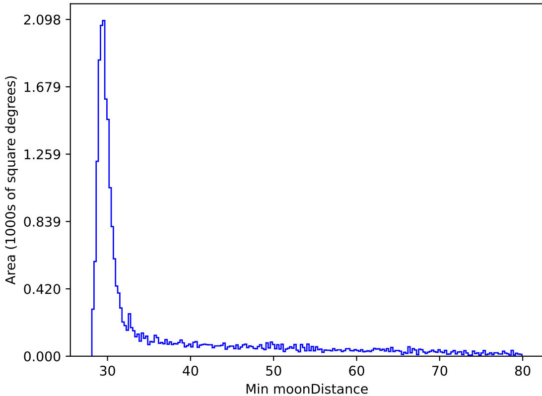
baseline_v3.3_10yrs All sky y band: Min moonDistance
