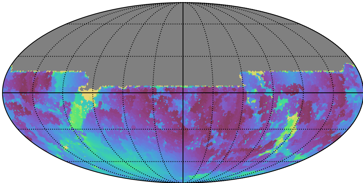
baseline_v3.3_10yrs All sky u band: Min moonDistance
