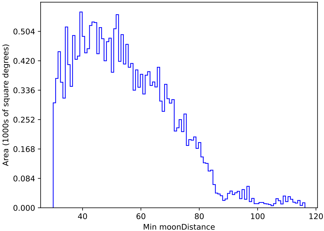
baseline_v3.3_10yrs All sky u band: Min moonDistance
