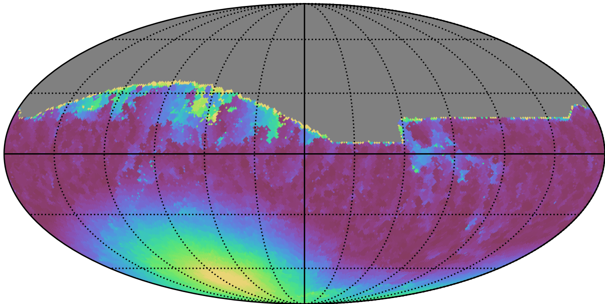
baseline_v3.3_10yrs All sky r band: Min moonDistance
