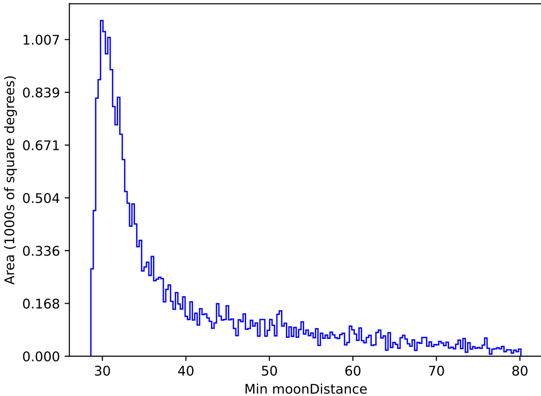
baseline_v3.3_10yrs All sky r band: Min moonDistance
