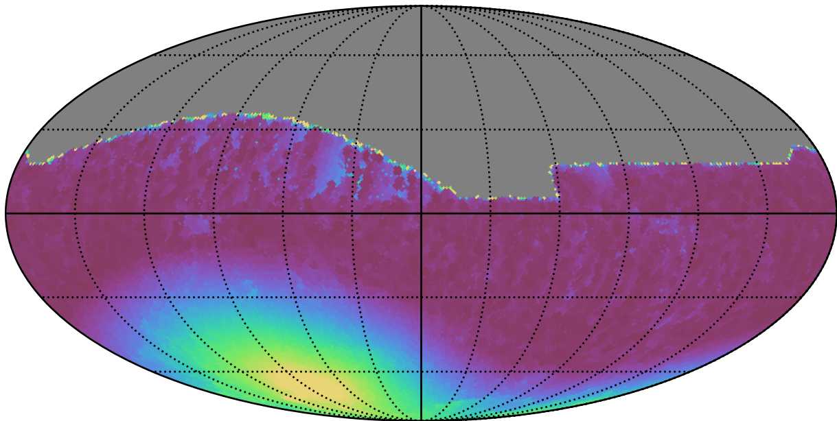
baseline_v3.3_10yrs All sky i band: Min moonDistance
