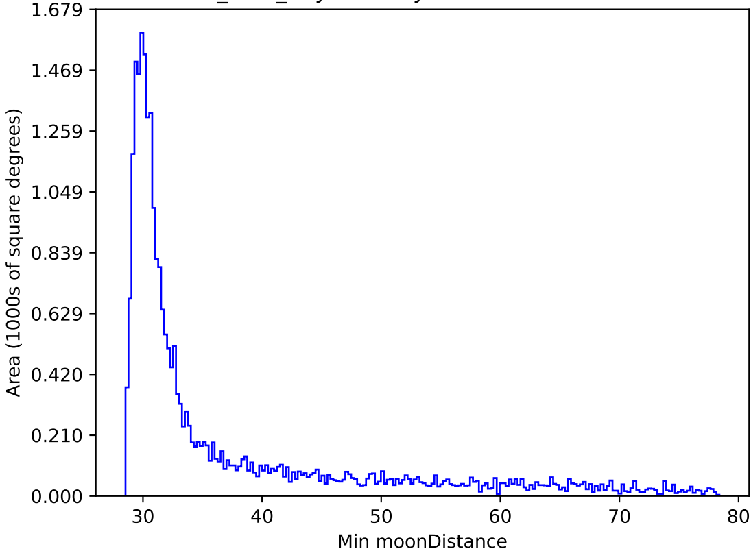
baseline_v3.3_10yrs All sky i band: Min moonDistance
