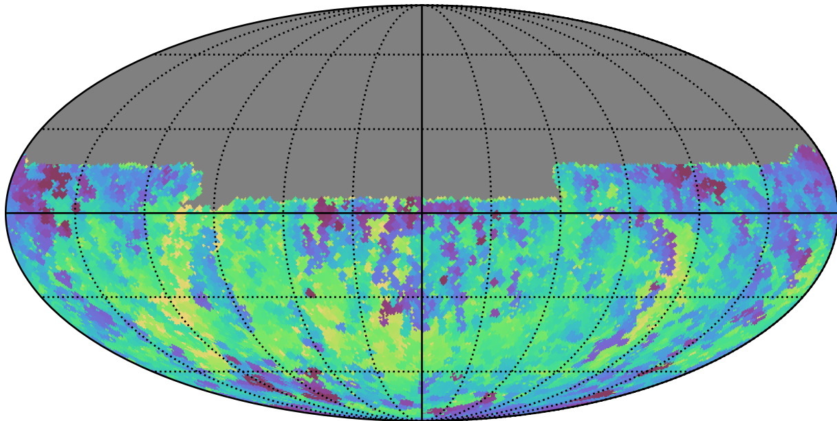
baseline_v3.3_10yrs Yr 1 y band: Min fiveSigmaDepth
