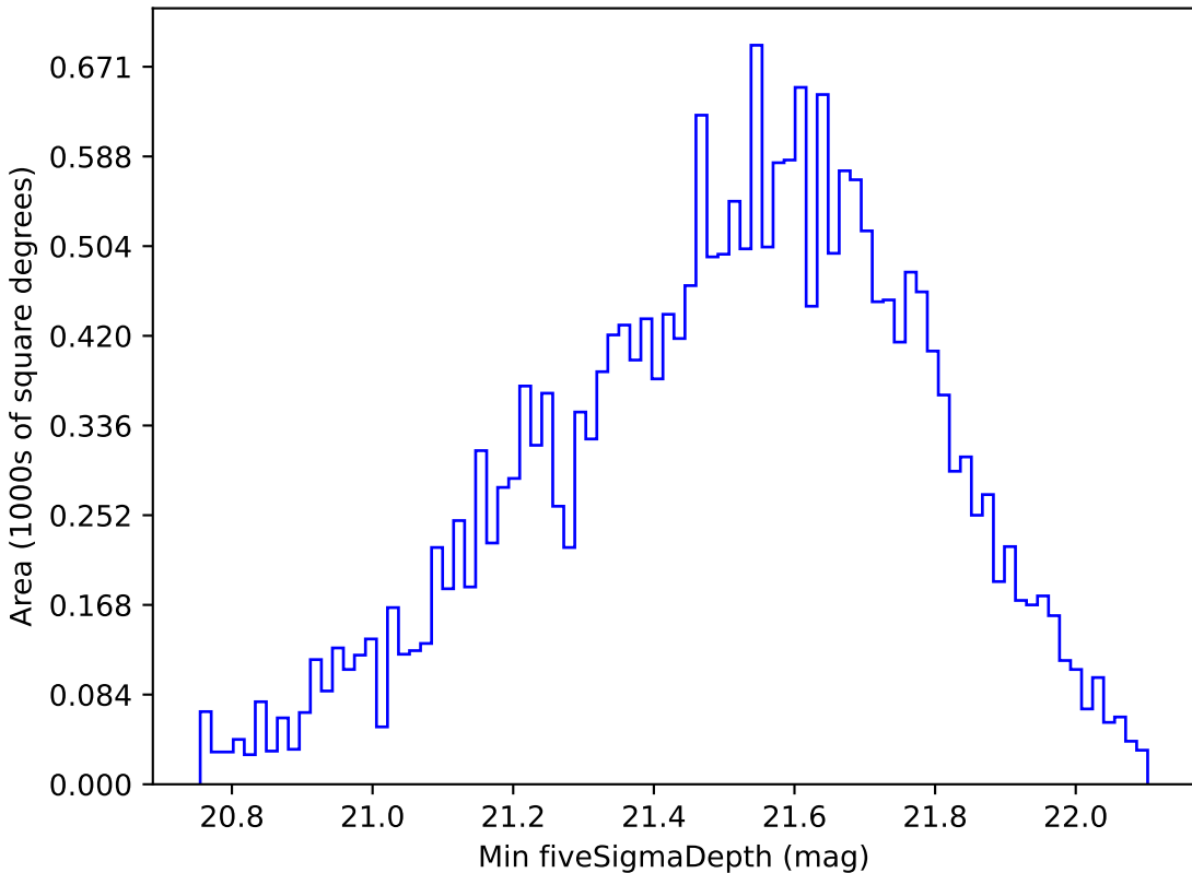
baseline_v3.3_10yrs Yr 1 y band: Min fiveSigmaDepth
