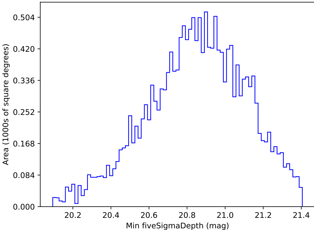
baseline_v3.3_10yrs WFD y band: Min fiveSigmaDepth
