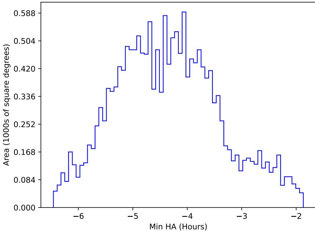
baseline_v3.3_10yrs WFD z band: Min HA
